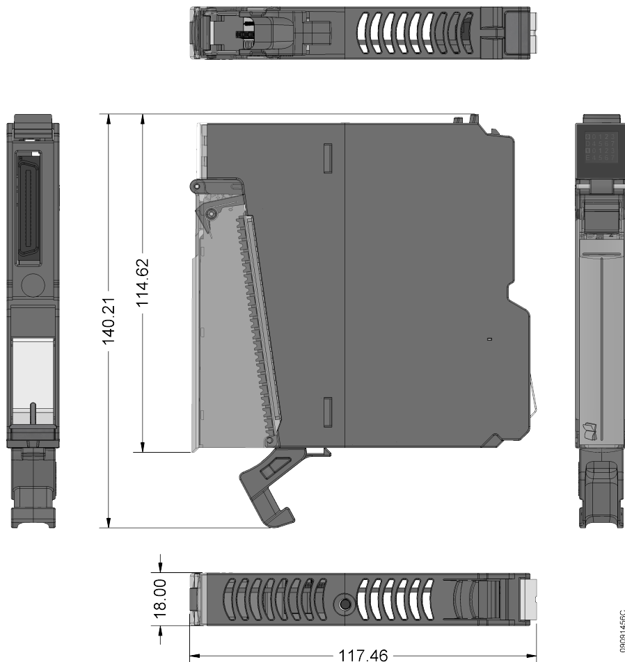
Figura 1: Dimensões Físicas
