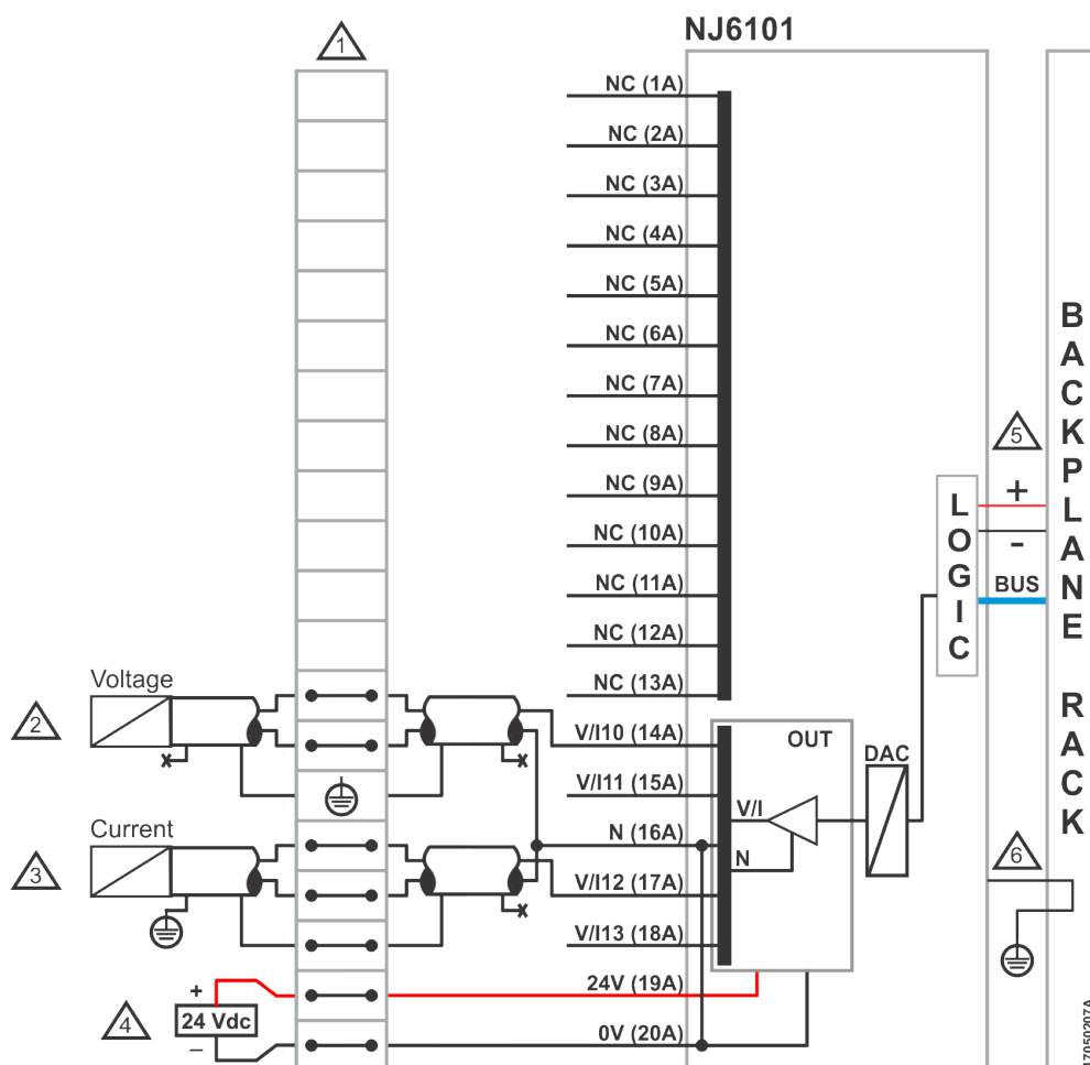
Figura 3: Diagrama Elétrico
