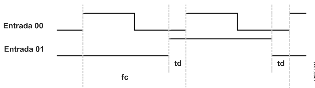
Figura 6: Contador
