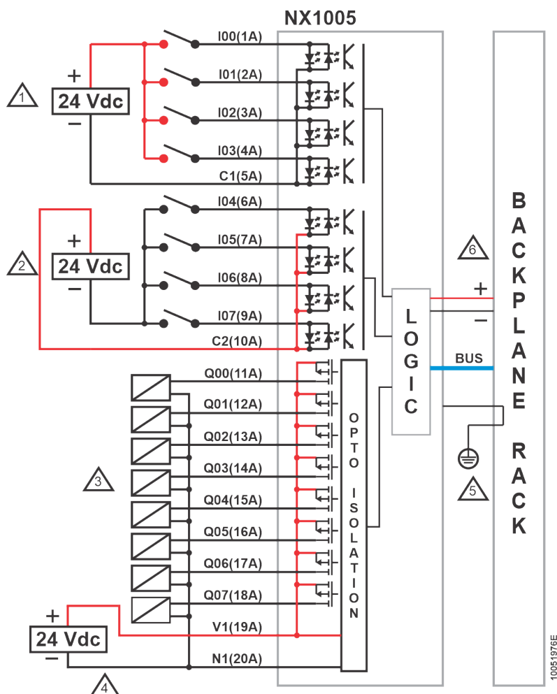
Figura 3: Diagrama Elétrico
