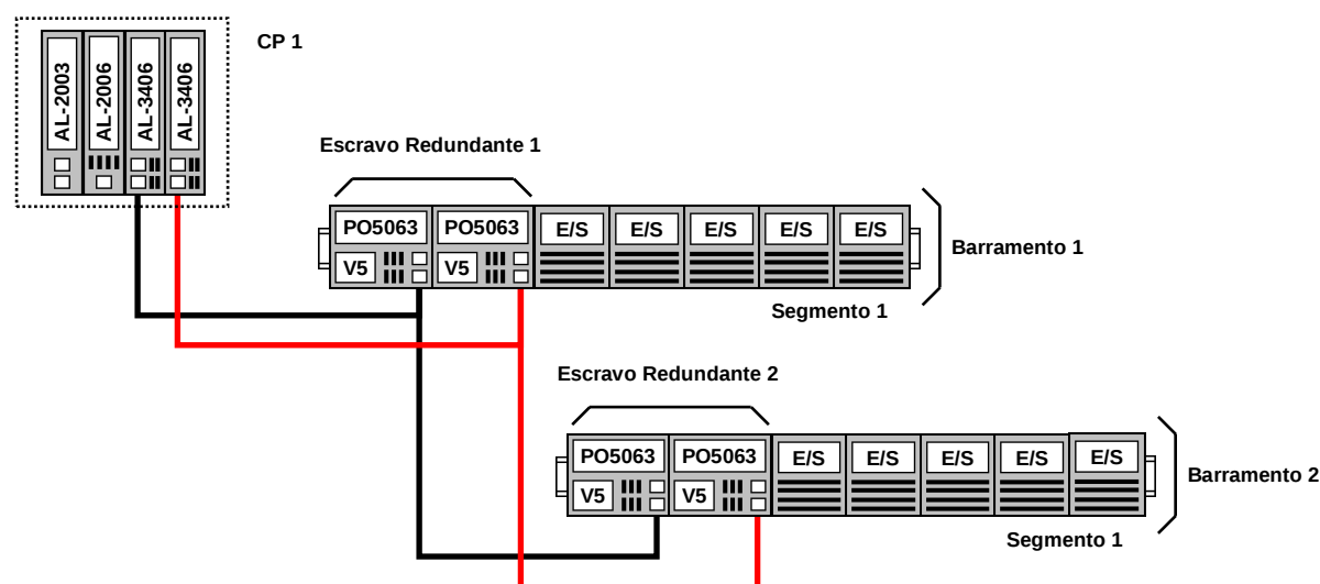
Figura 12-4 Sistema Redundante de Meio Físico e Mestre Utilizando AL-3406
