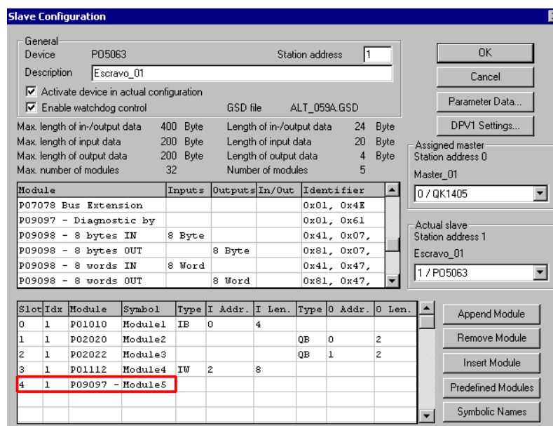
Figura 10-1 Declaração da IHM na rede PROFIBUS
