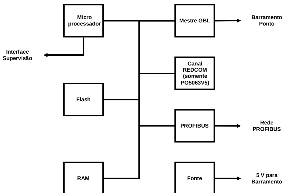
Figura 2-4 Diagrama de Blocos da PO5063V1 e PO5063V5
