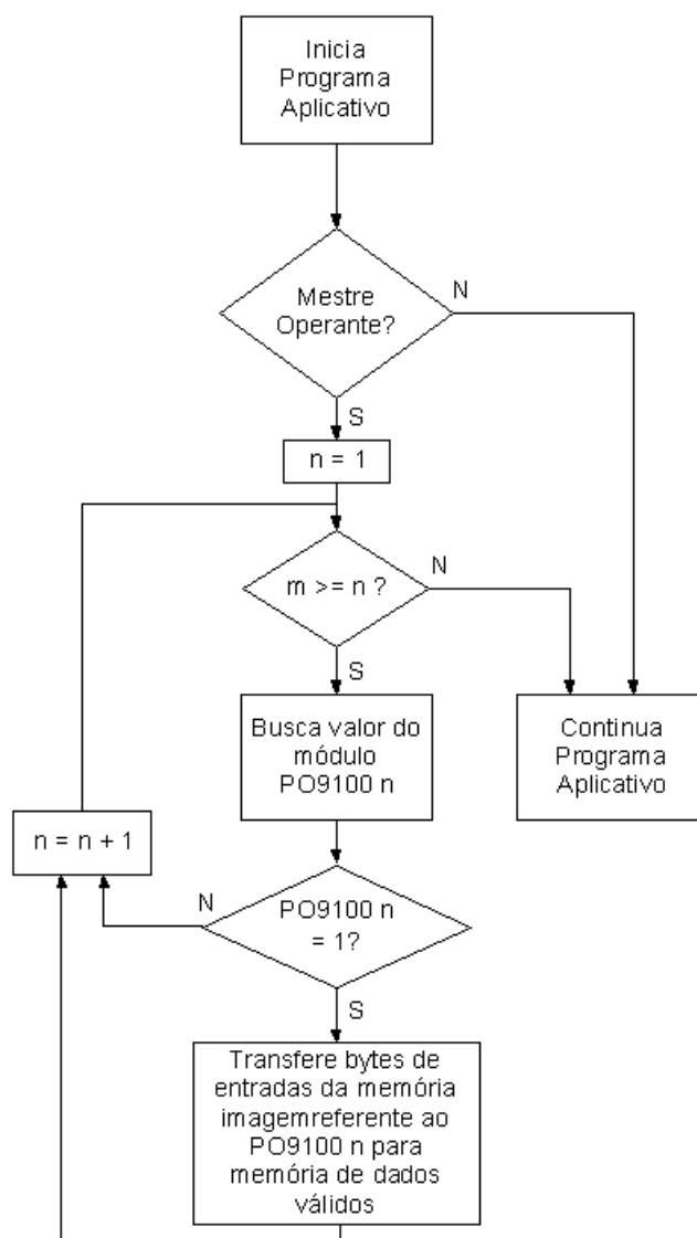
Figura 11.1 – Algoritmos de Redundância a Nível de Dispositivo Mestre
