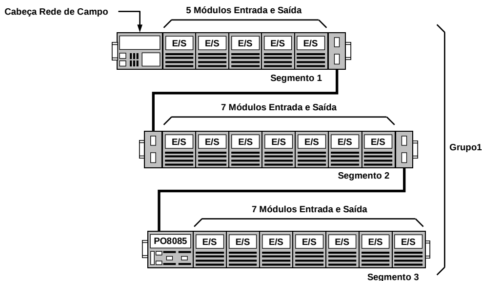
Figura 4-2 Exemplo 1 Utilizando Três Segmentos
