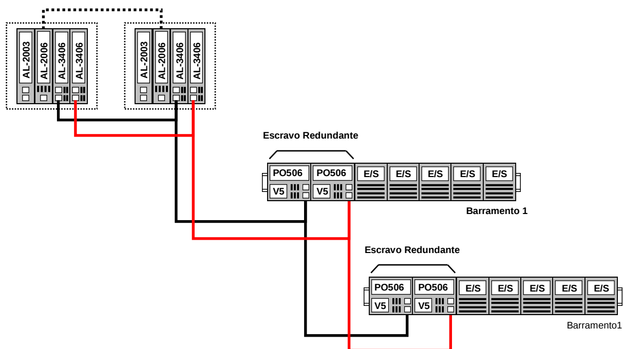
Figura 12-7 Sistema Redundante Completo
