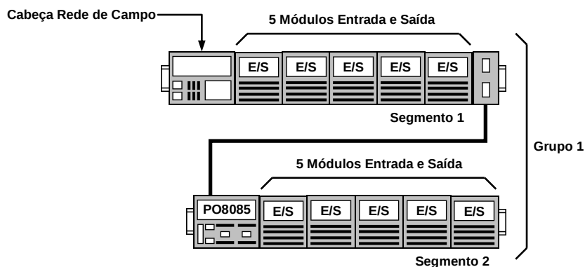
Figura 4-3 Exemplo 2 Utilizando Dois Segmentos
