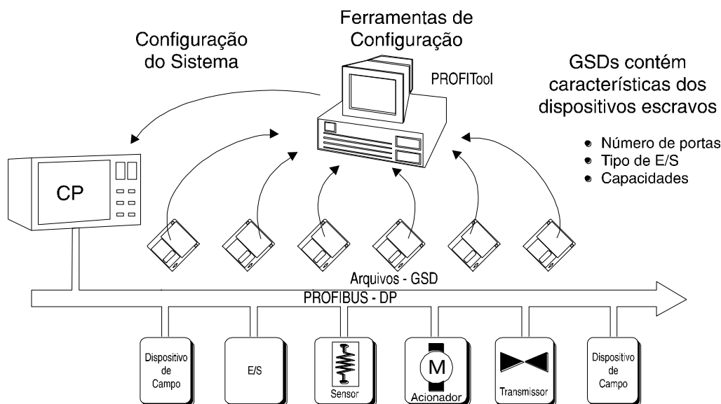
Figura 2-5 Configuração através de Arquivos GSD
