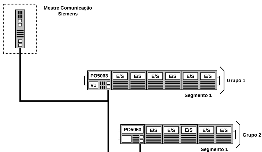
Figura 4-13 Cabeças PROFIBUS e Mestre Siemens
