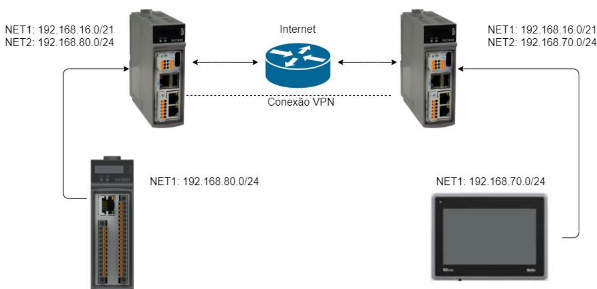
Figura 184: Exemplo de Arquitetura com Redes Privadas
