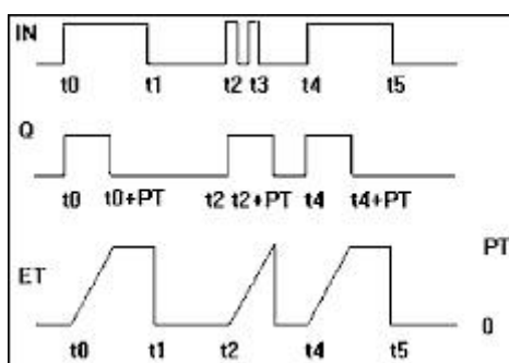
Figura 170: Comportamento Gráfico do Bloco Funcional TP_RET
