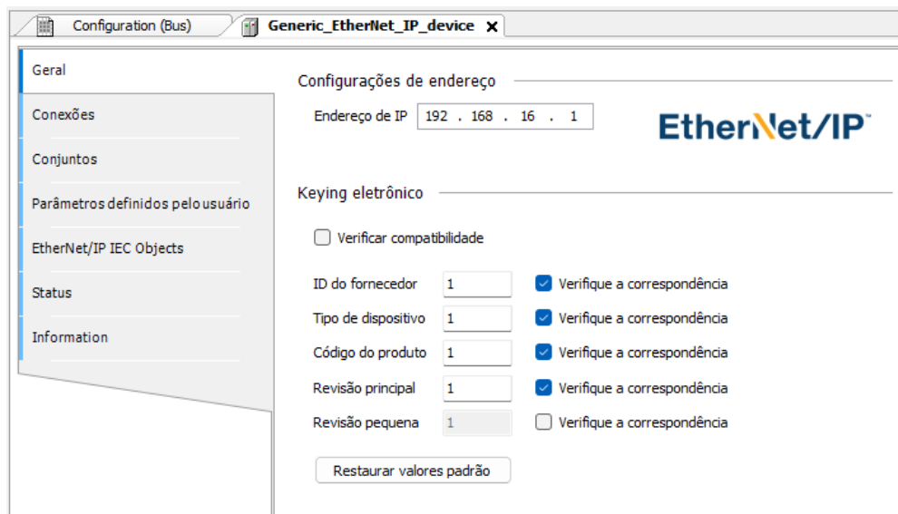
Figura 120: Aba Geral - EtherNet/IP
