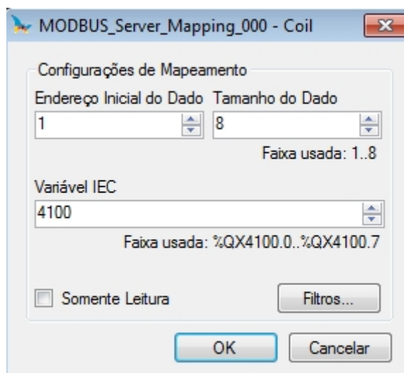
Figura 97: Função MODBUS Servidor
