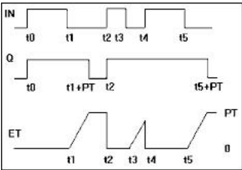
Figura 166: Comportamento Gráfico do Bloco Funcional TOF_RET
