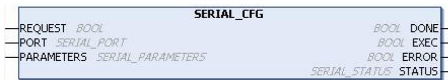
Figura 155: Bloco de Configuração da Serial
