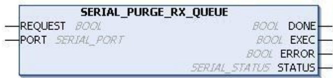
Figura 158: Bloco para Limpar a Fila RX
