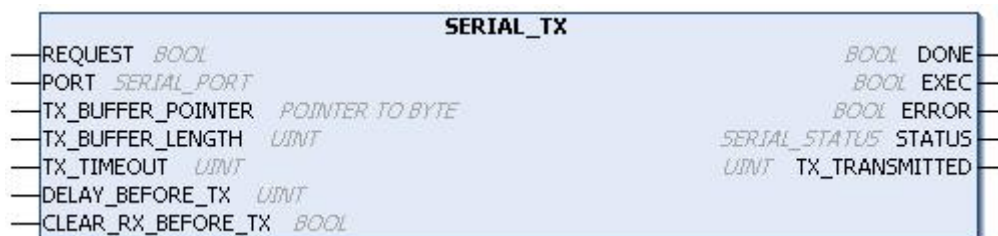
Figura 162: Bloco para Transmitir Valores pela SERIAL_TX
