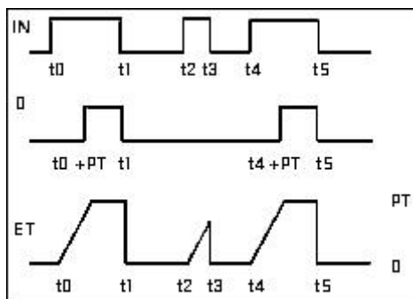
Figura 168: Comportamento Gráfico do Bloco Funcional TON_RET
