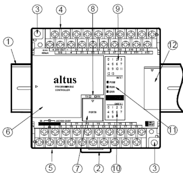
(vista frontal sem board de expansão)
