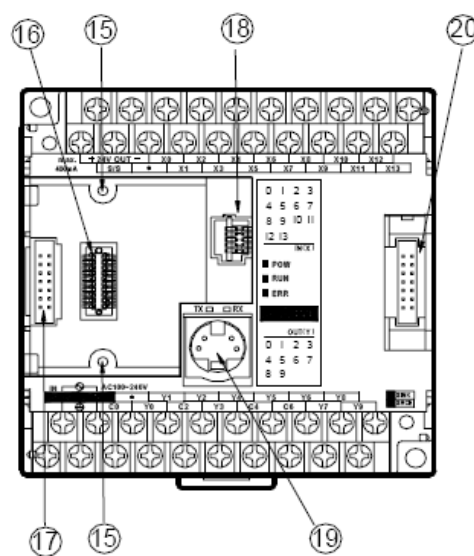
(vista frontal sem a tampa frontal)
