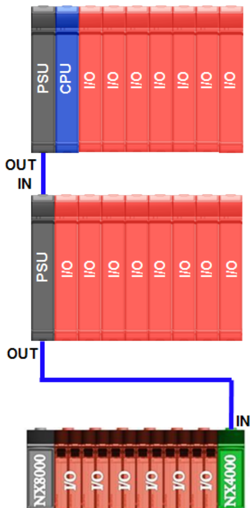
Figura 12: Expansão de barramento com Nexto
