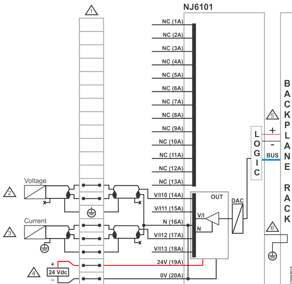
Figura 3: Diagrama Elétrico
