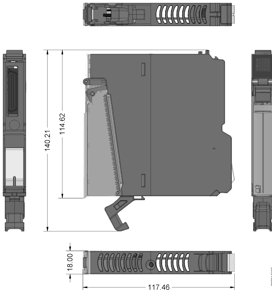
Figura 1: Dimensões Físicas
