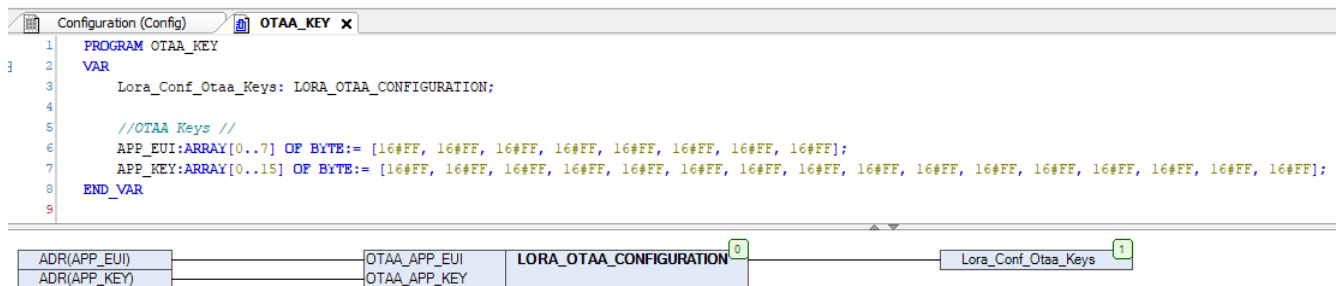
Figura 13: LORA_OTAA_CONFIGURATION
