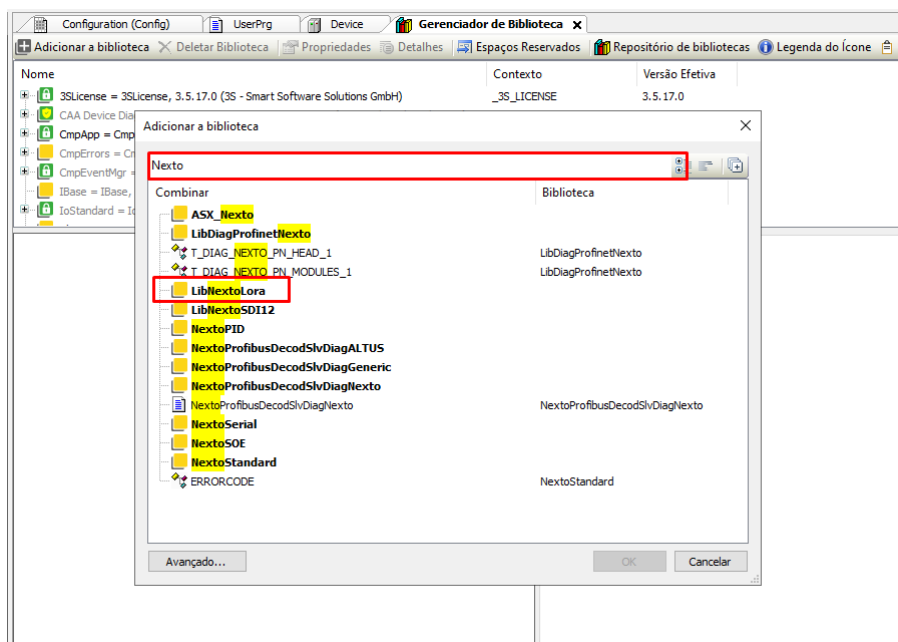
Figura 8: Biblioteca LibNextoLora
