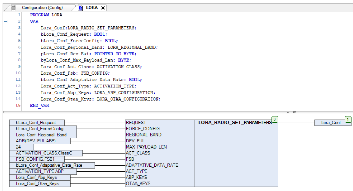
Figura 11: LORA_RADIO_SET_PARAMETERS
