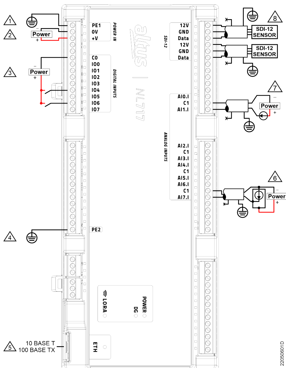
Figura 1: Diagrama de Instalação Elétrica
