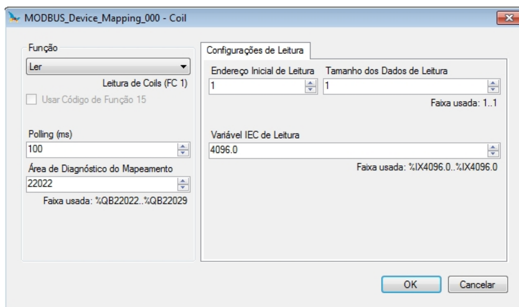
Figura 50: Função MODBUS
