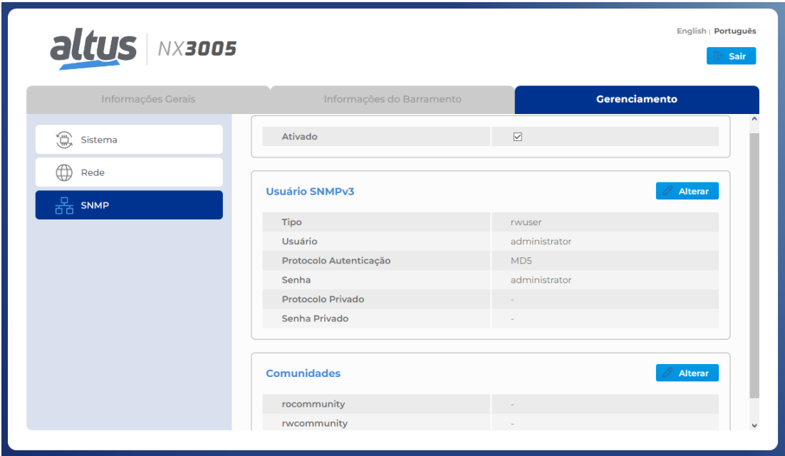
Figura 143: Tela de Configuração e Status SNMP
