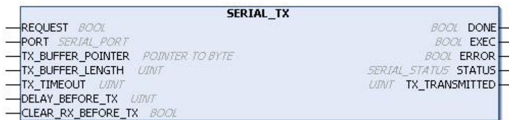
Figura 127: Bloco para Transmitir Valores pela SERIAL_TX
