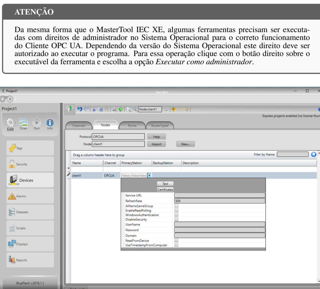
Figura 87: Selecionando Servidor OPC UA na Configuração do Cliente
