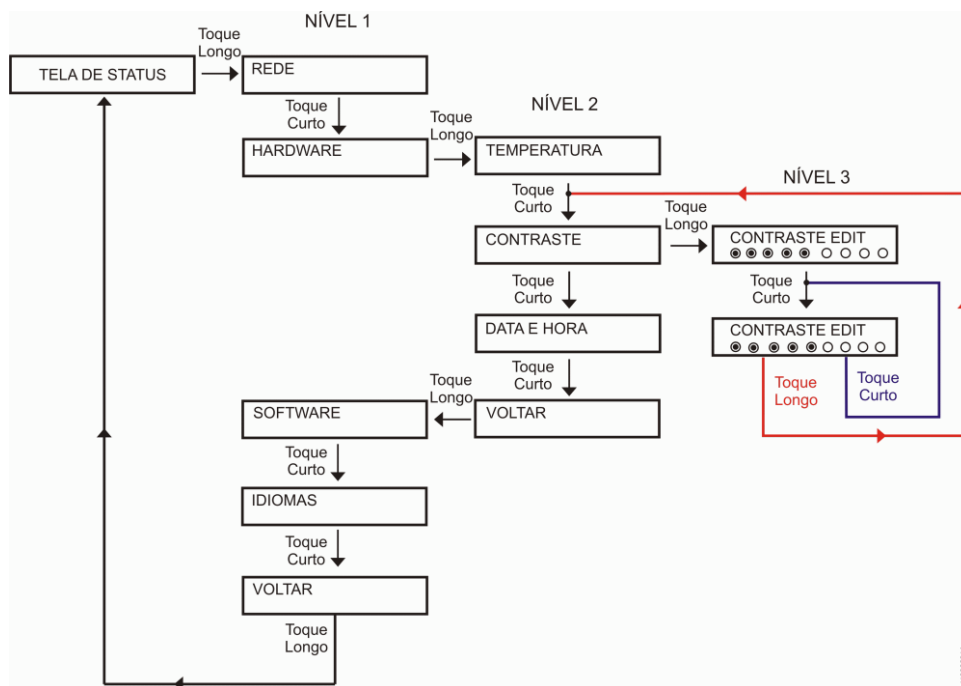
Figura 118: Ajuste do Contraste
