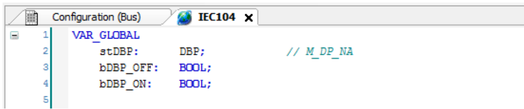
Figura 99: Exemplo de Declaração das Variáveis de Ponto Duplo
