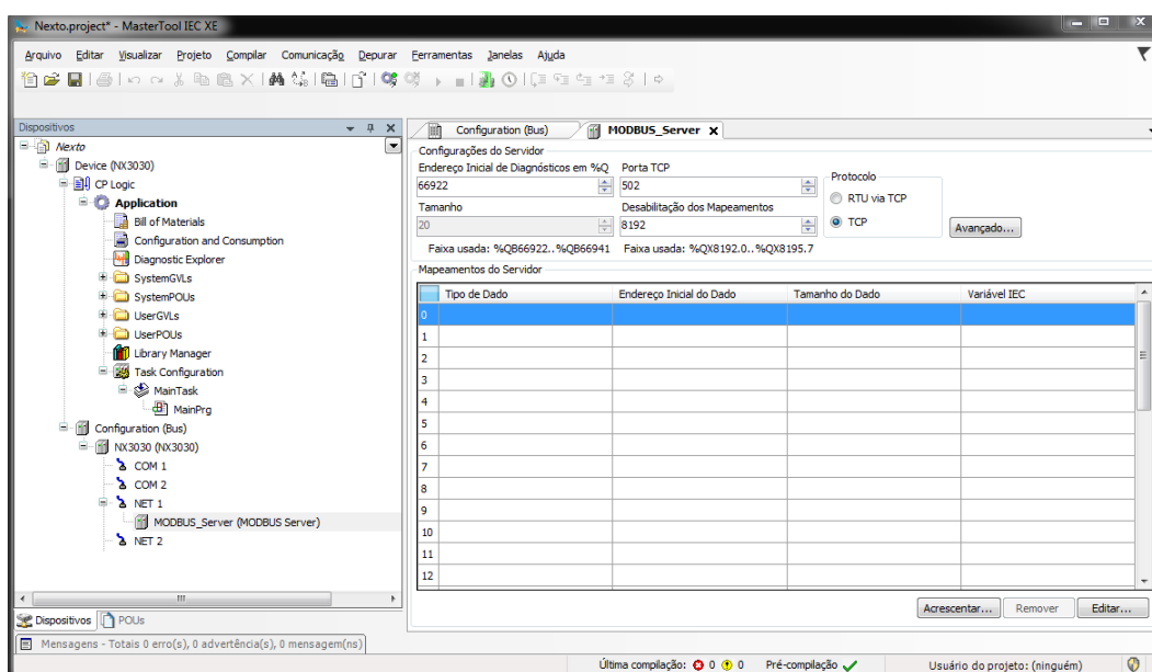
Figura 75: Tela de Configuração MODBUS Servidor
