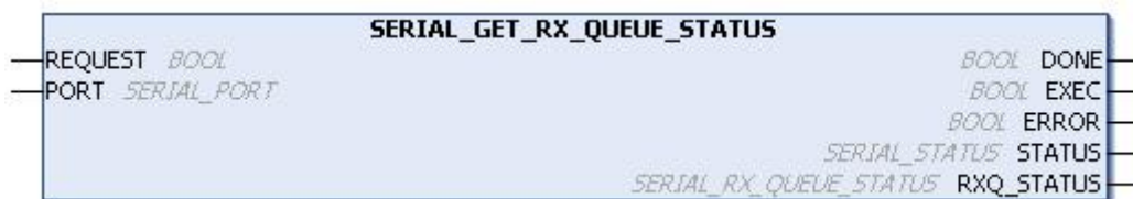
Figura 122: Bloco para Visualizar o Status da Fila RX
