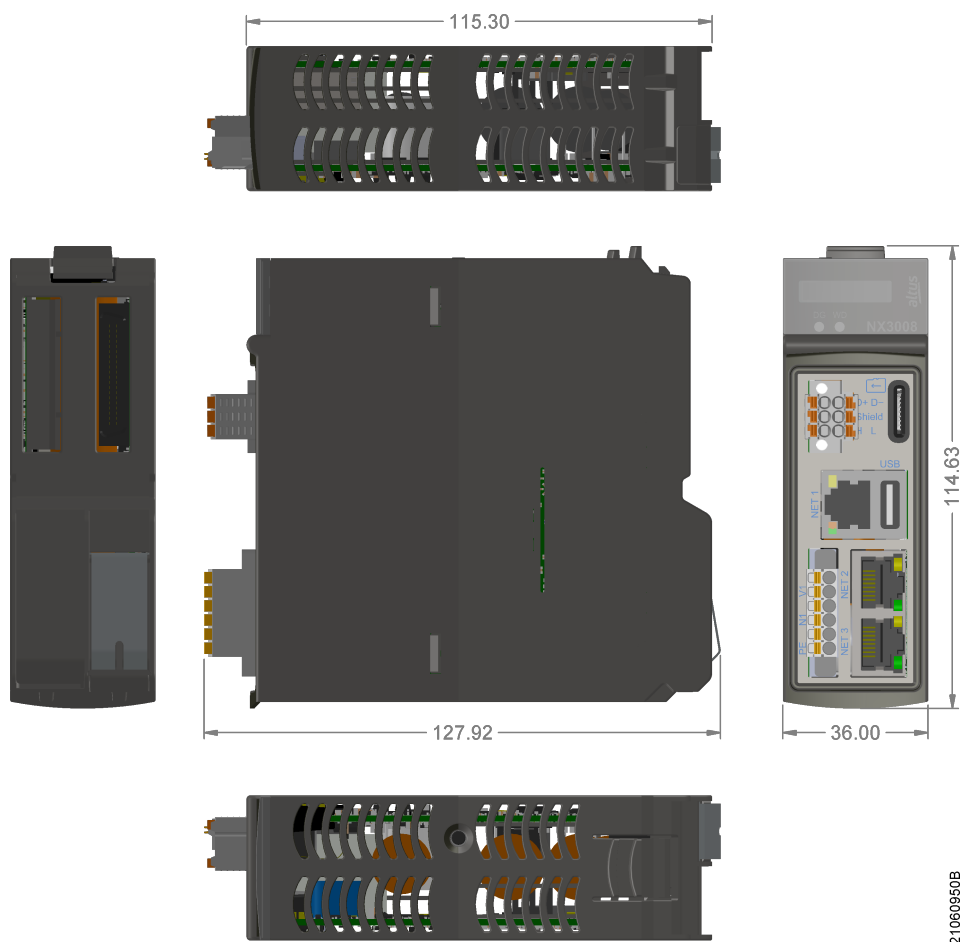
Figura 1: Dimensões Físicas
