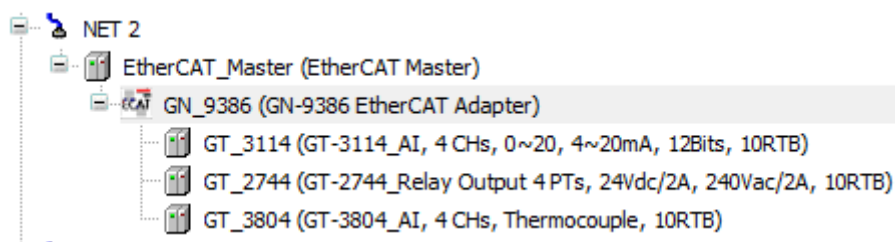
Figura 93: Exemplo de Configuração EtherCAT
