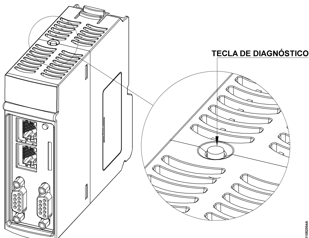
Figura 183: Tecla de Diagnóstico
