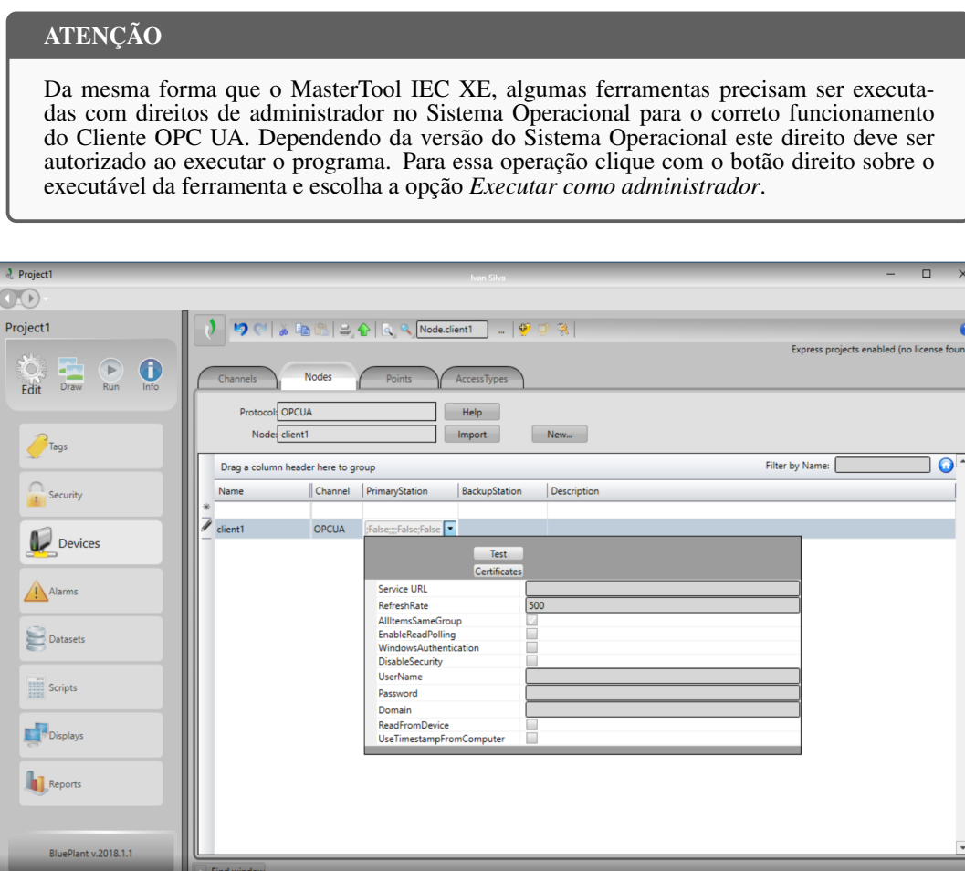
Figura 91: Selecionando Servidor OPC UA na Configuração do Cliente
