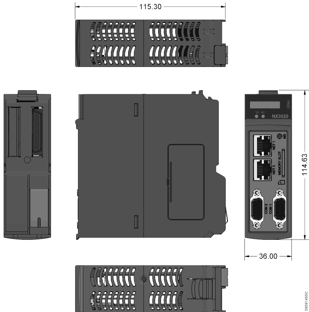
Figura 4: Dimensões Físicas
