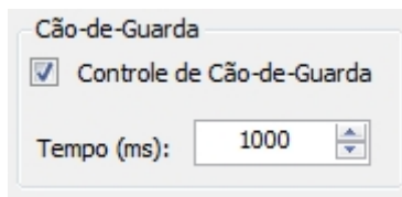
Figura 180: Configuração de Cão-de-Guarda de uma Remota PROFIBUS
