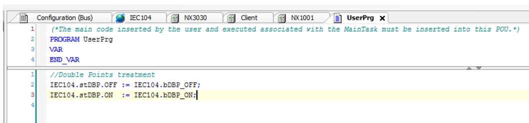
Figura 115: Atribuição dos Valores das Variáveis ao Ponto Duplo
