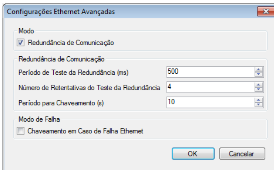
Figura 178: Configurações Avançadas da Ethernet
