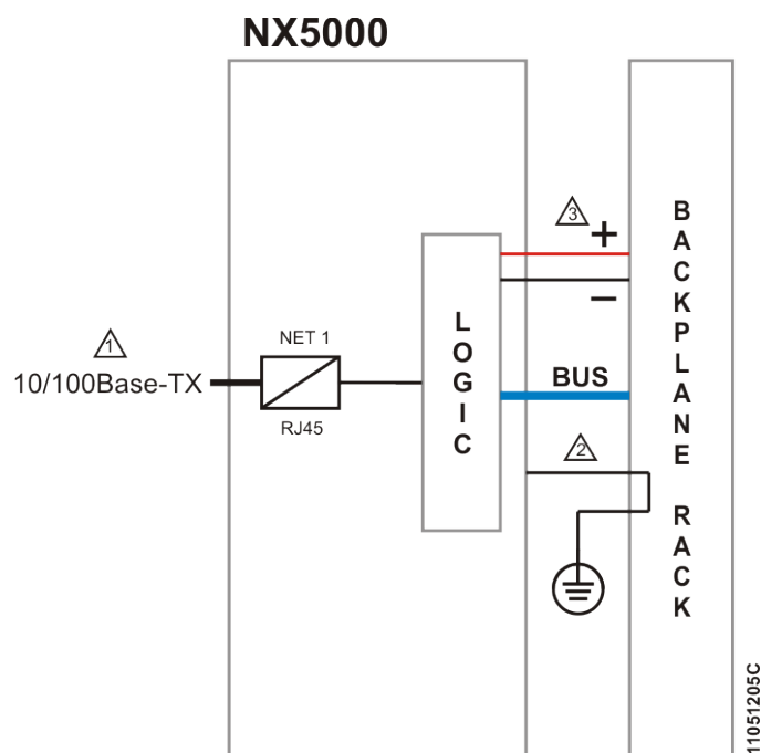
Figura 3: Diagrama Elétrico
