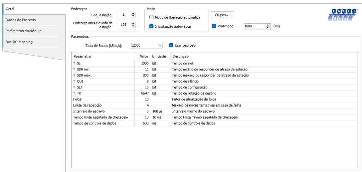
Figura 18: Parametrização do Barramento PROFIBUS
