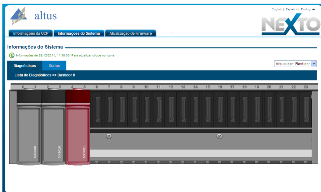
Figura 11: Página Web
