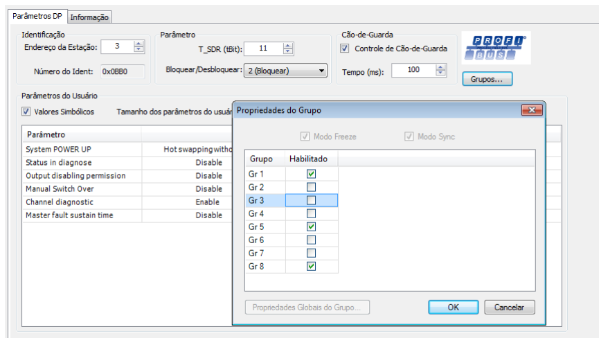
Figura 29: Configuração de Grupo do Escravo PROFIBUS
