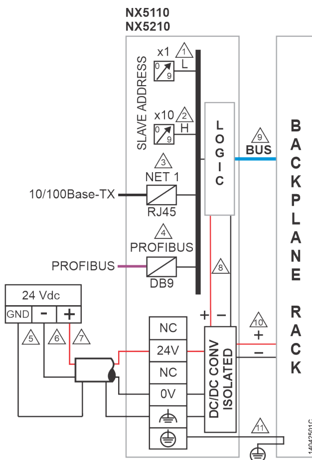
Figura 6: Diagrama Elétrico
