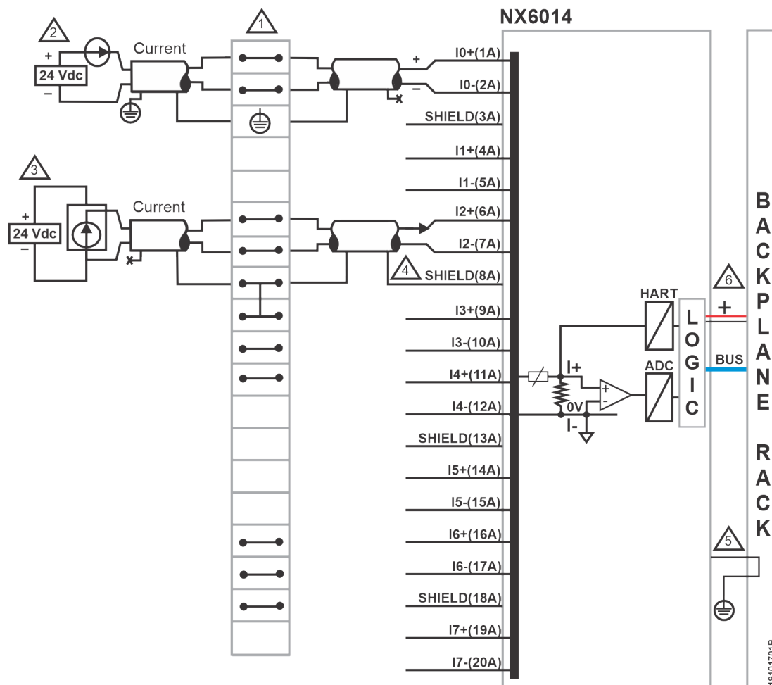
Figura 3: Diagrama Elétrico
