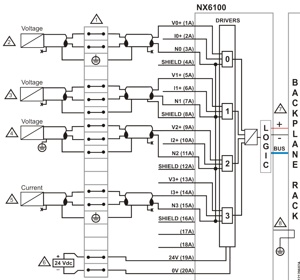
Figura 3: Diagrama Elétrico
