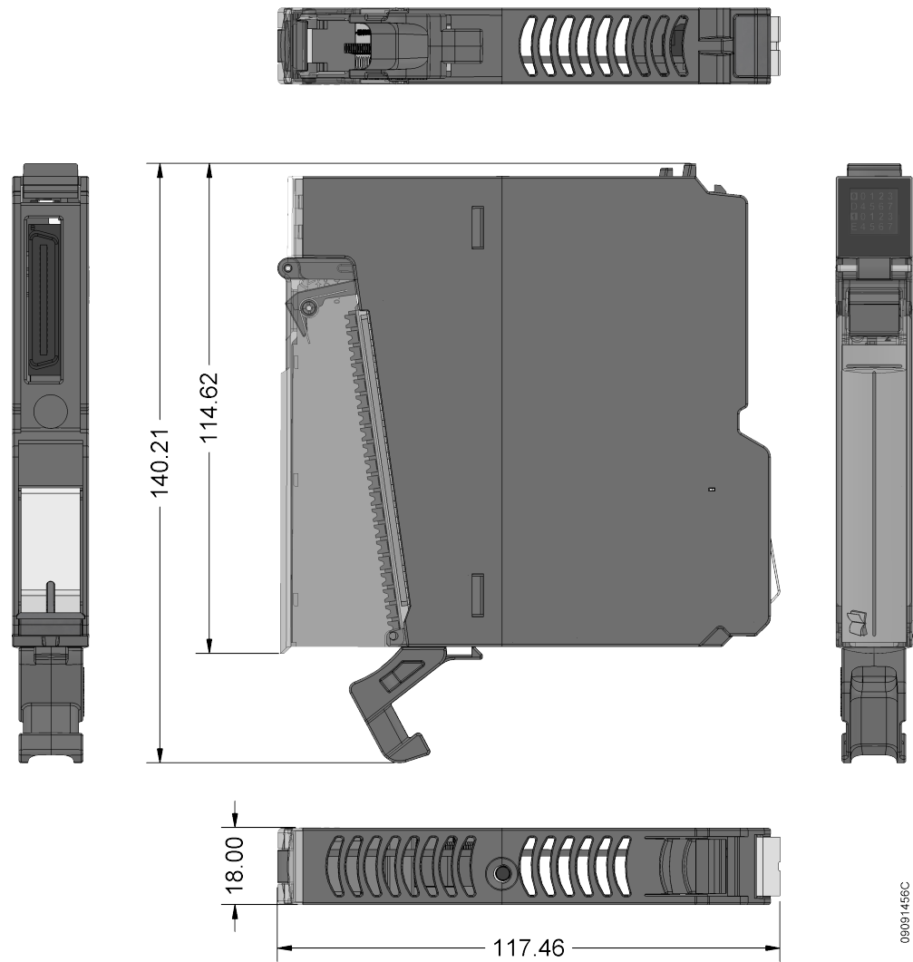
Figura 1: Dimensões Físicas
