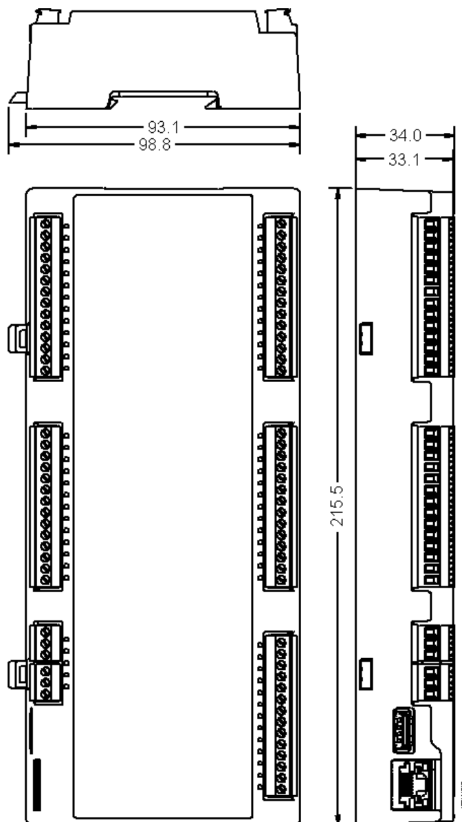
Figura 2: Dimensões Físicas do XP3xx
