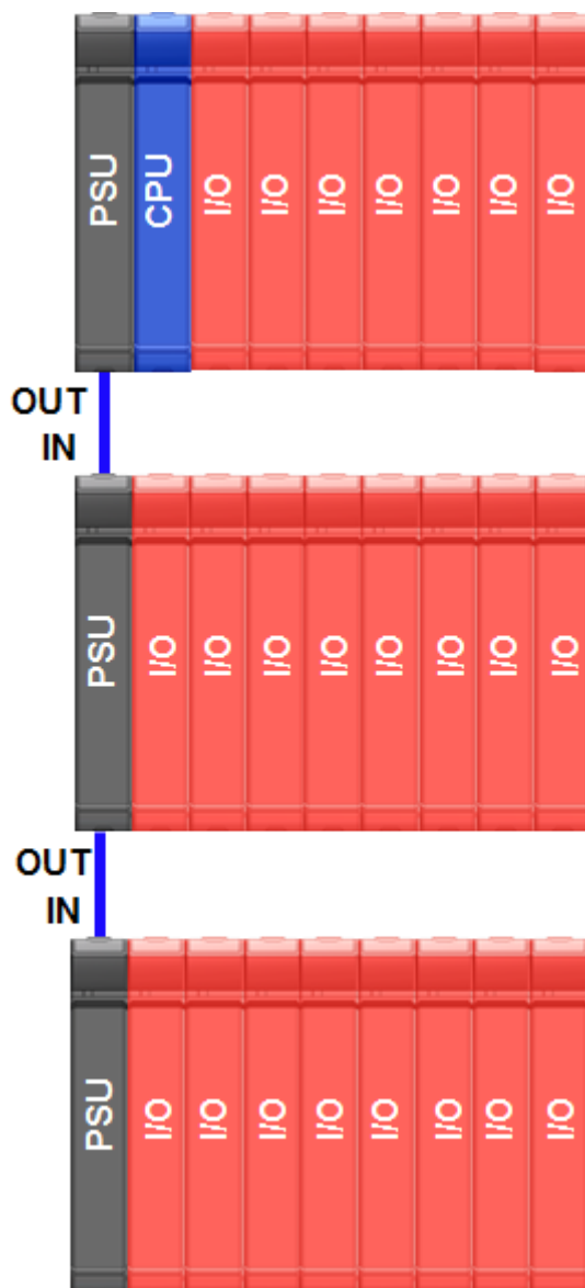
Figura 4: UCP com E/S Remoto (Expansão de Barramento)
