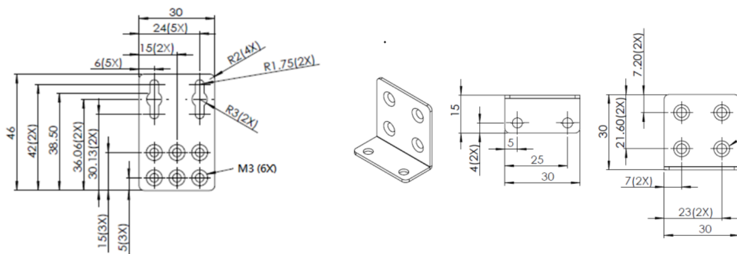
Figura 36: Dimensões do suporte para montagem em parede
