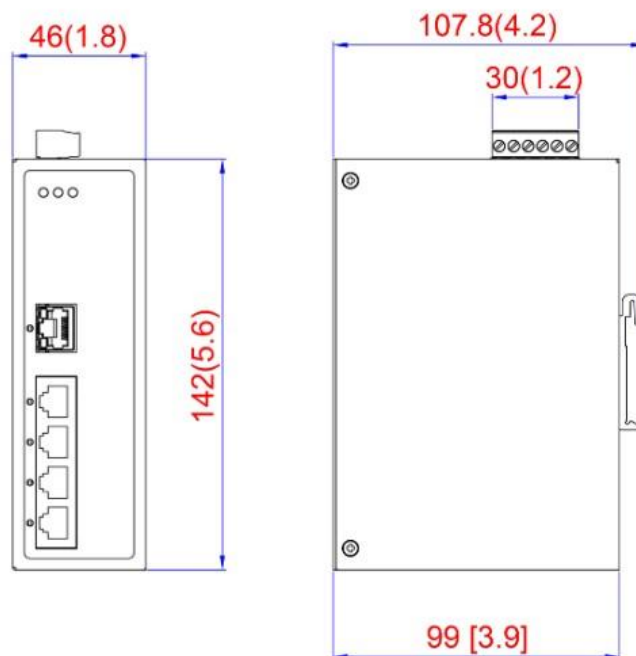
Figura 16: Dimensões Físicas do PT2-0500-24
