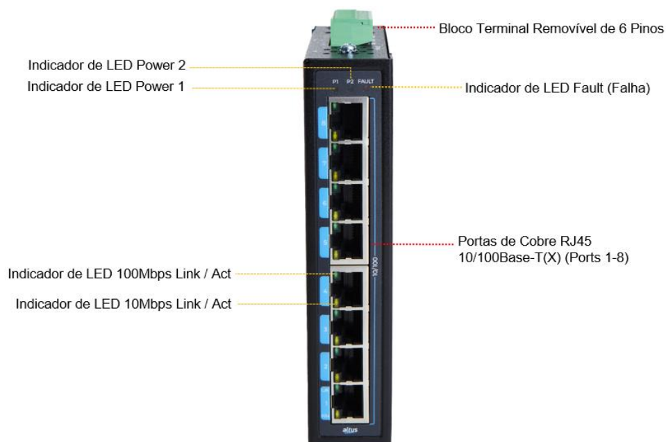
Figura 5: Painel Frontal do ET2-0800
