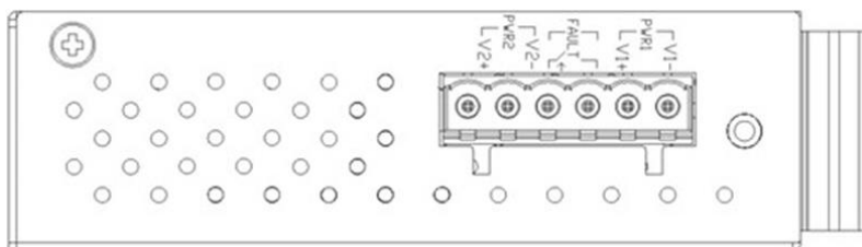
Figura 9: Visão do Painel Superior do ET2-0602-M
