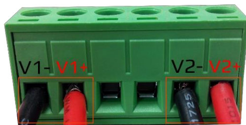
Figura 25: Bloco Terminal de Alimentação
