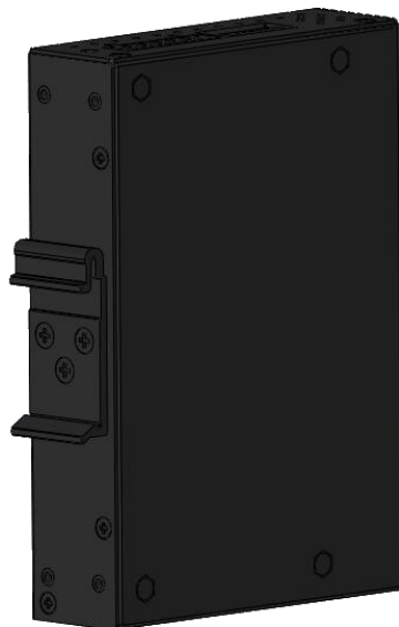
Figura 31: Parte traseira do switch e suporte para trilho DIN
