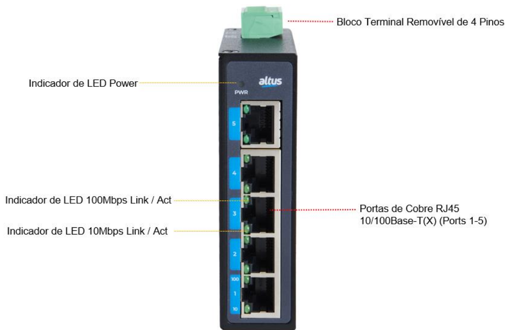
Figura 2: Pannel Frontal do CET2-0500
