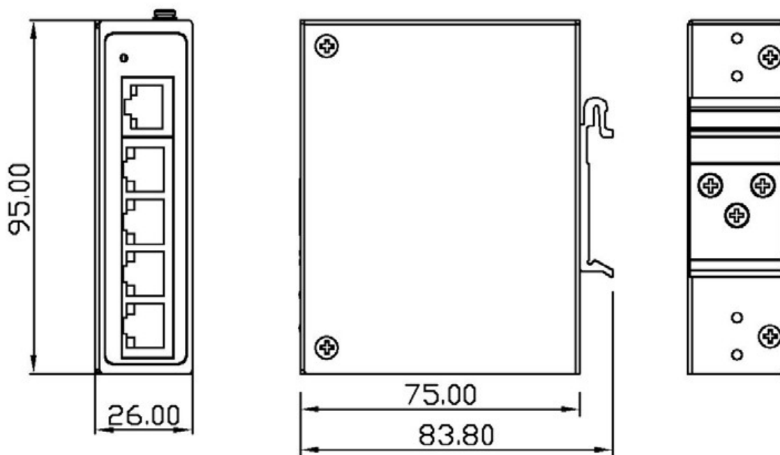
Figura 1: Dimensões Físicas do CET2-0500
