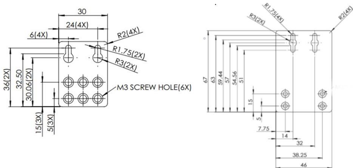
Figura 37: Dimensões do suporte para montagem em parede
