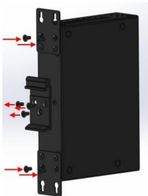
Figura 35: Suporte para montagem de parede
