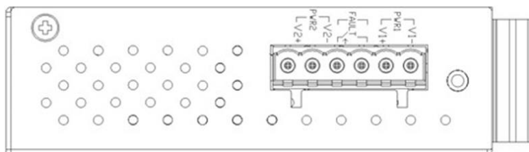
Figura 12: Visão do Painel Superior do ET2-1600
