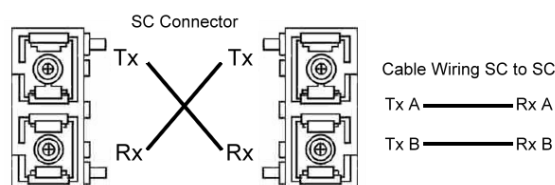
Figura 19: Porta Fibra do conector SC Multimodo
