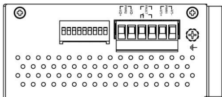
Figura 18: Visão do Painel Superior do PT2-0500-24
