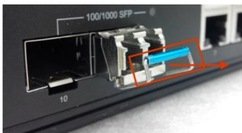
Figura 24: Retirar do módulo SFP
