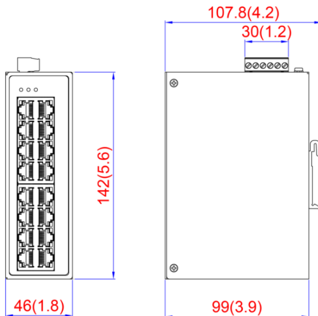
Figura 10: Dimensões Físicas do ET2-1600
