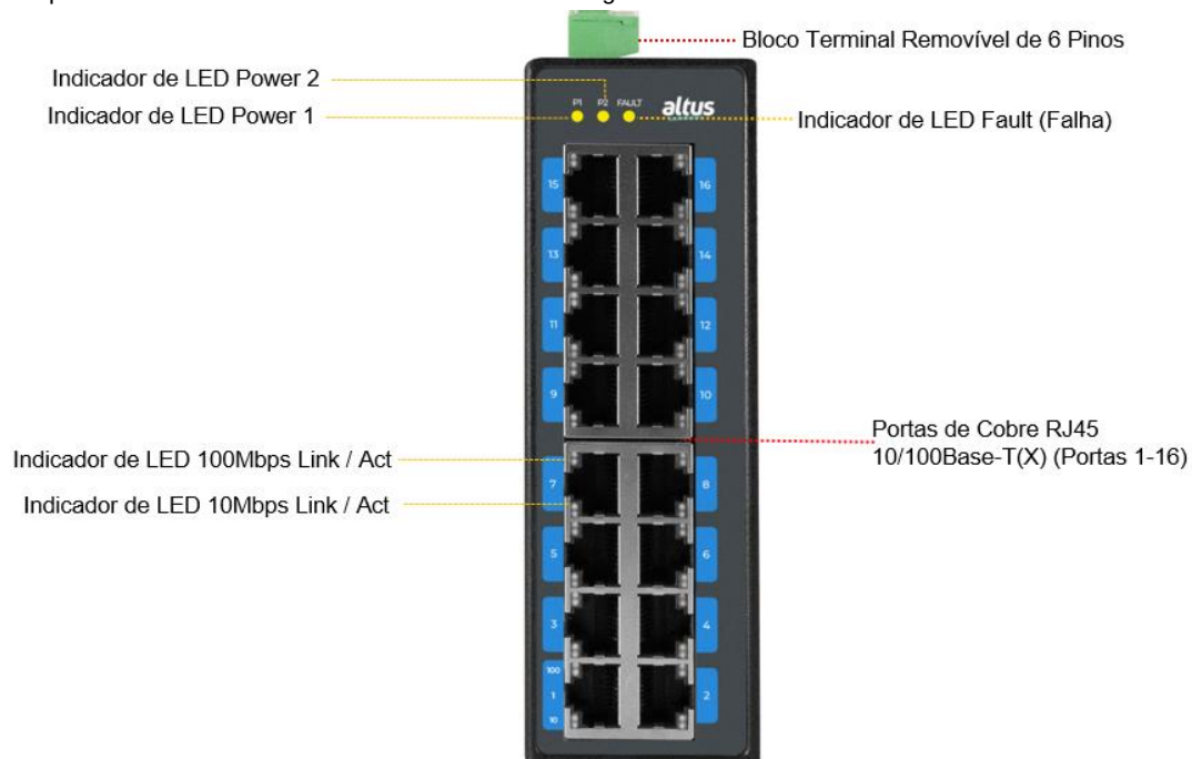
Figura 11: Painel Frontal do ET2-1600
