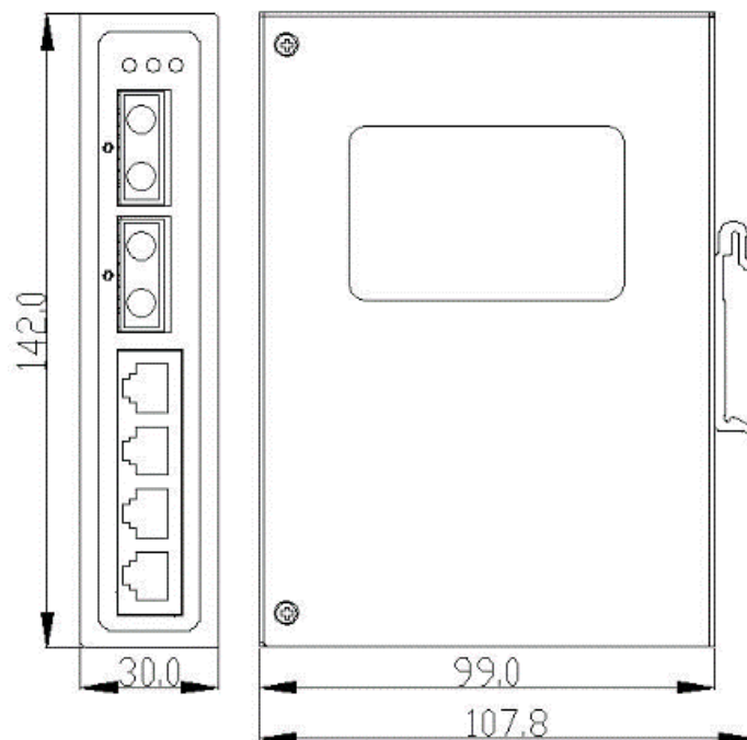
Figura 7: Dimensões Físicas do ET2-0602-M
