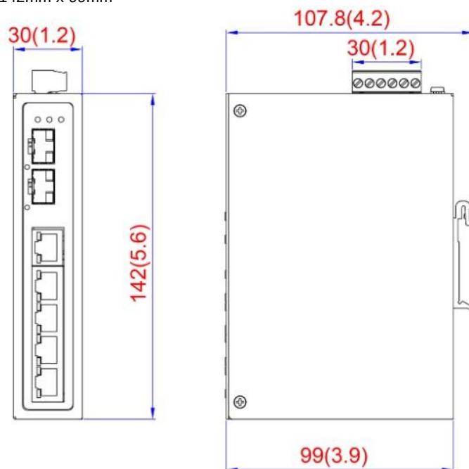
Figura 13: Dimensões Físicas do ET2-0702-SFP
