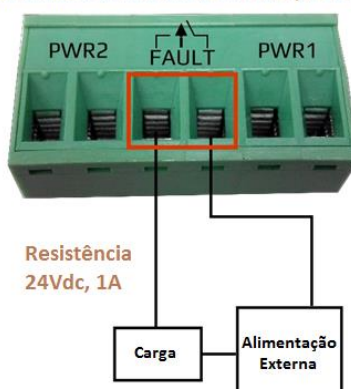
Figura 30: Conectando o Contato de Alarme Fault nos Switches ET2-0800, ET2-0602-M, ET2-1600, ET2-0702-SFP and PT2-0500-24
