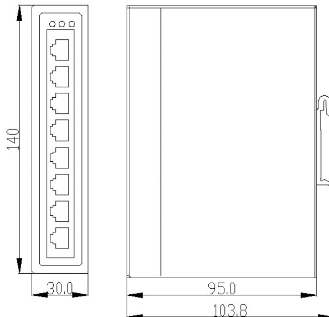
Figura 4: Dimensões Físicas do ET2-0800
