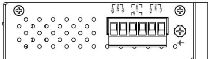
Figura 15: Visão do Painel Superior do ET2-0702-SFP
