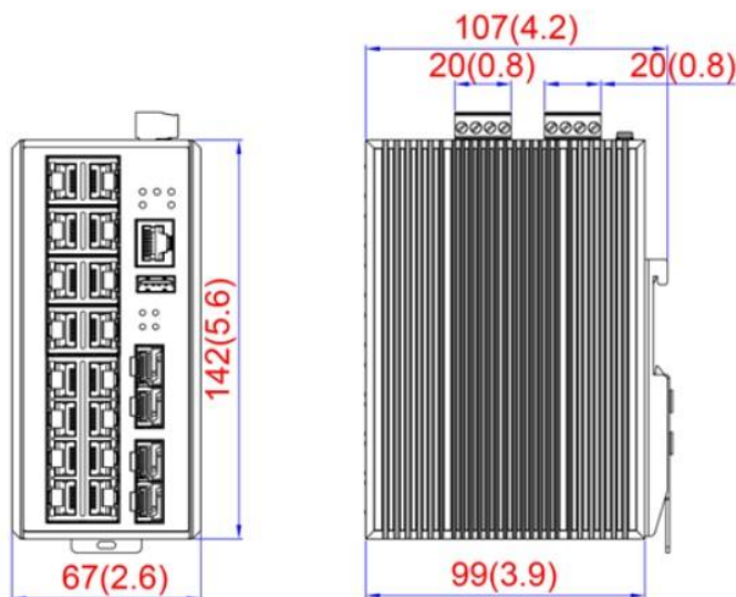
Figura 19: Dimensões Físicas do EG5-2004-SFP
