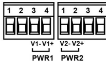
Figura 29: Bloco de terminais de energia
