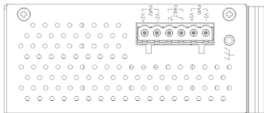
Figura 6: Visão do Painel Superior do ET5-0600
