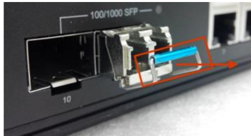
Figura 26: Retirar do módulo SFP
