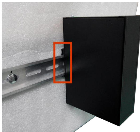
Figura 35: Estabilize o switch no trilho DIN
