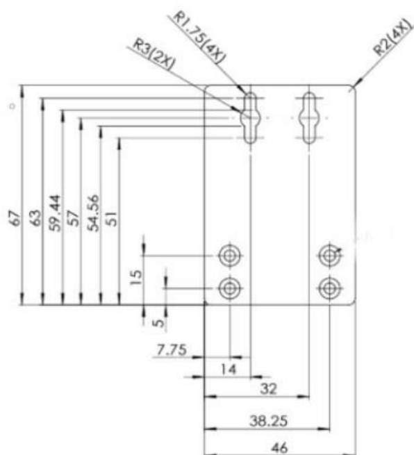
Figura 37: Dimensões do suporte para montagem em parede
