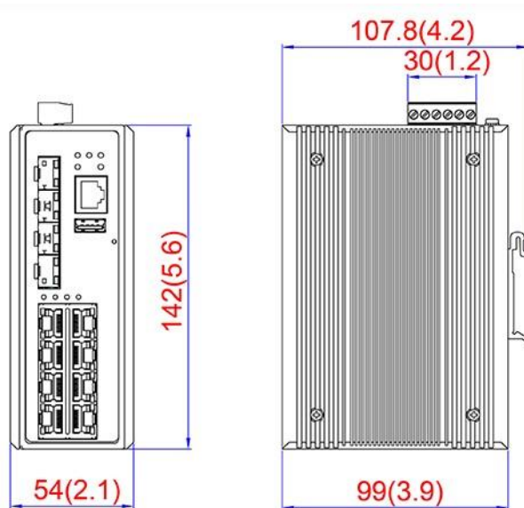
Figura 16: Dimensões Físicas do PG5-1204-SFP
