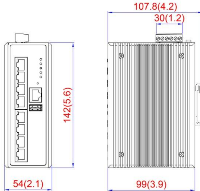
Figura 13: Dimensões Físicas do ET5-0800
