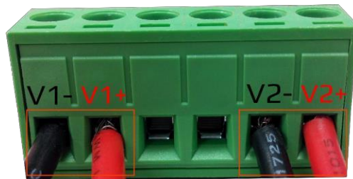
Figura 27: Bloco Terminal de Alimentação
