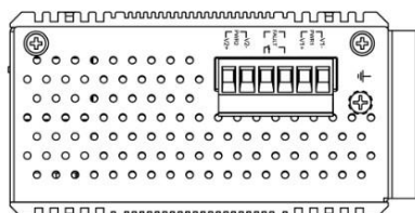
Figura 15: Visão do Painel Superior do ET5-0800
