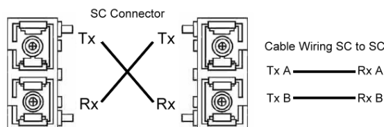
Figura 22: Porta Fibra do conector SC Multimodo
