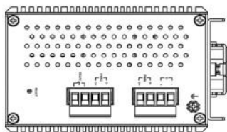
Figura 21: Visão do Pannel Superior do EG5-2004-SFP
