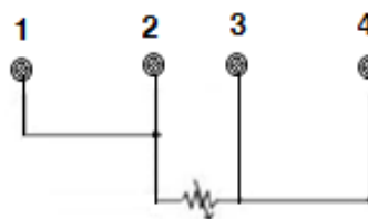
Conexão RTD ou resistivo diferencial, máximo, mínimo e backup.
