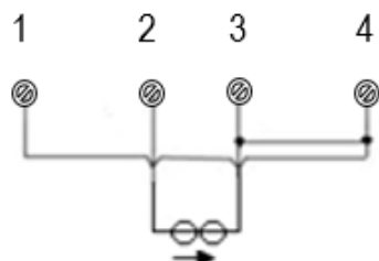
Conexão entrada 4 – 20 mA.
