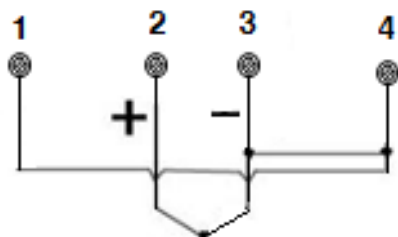
Conexão termopar ou mV
