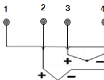
Conexão termopar ou mV diferencial, máximo, mínimo e backup
