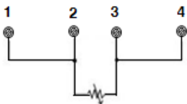
Conexão RTD ou resistivos a 4 fios.
