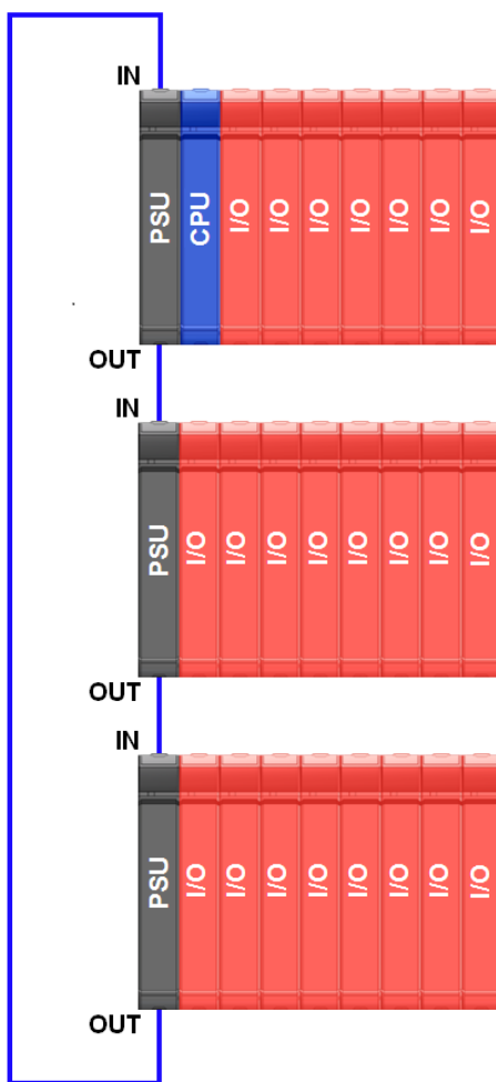
Figura 3: Expansão de Barramento com Loopback
