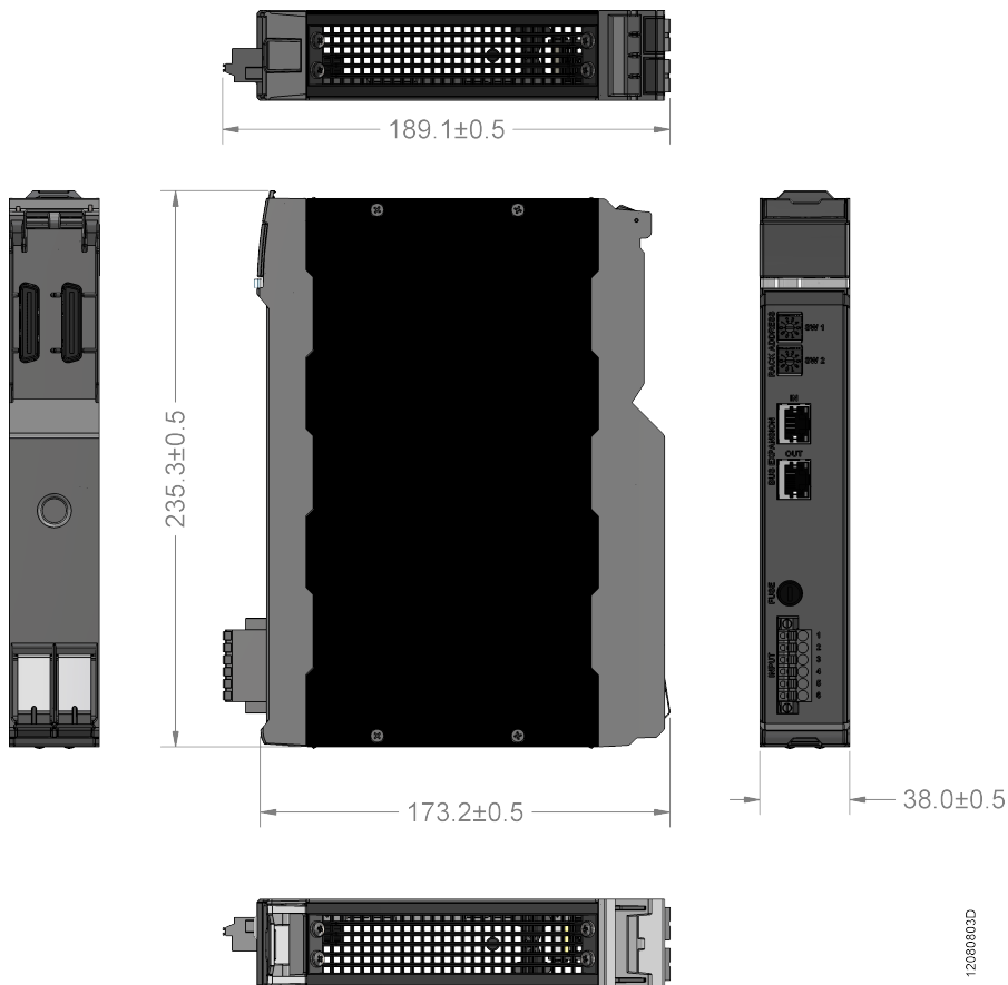
Figura 5: Dimensões Físicas
