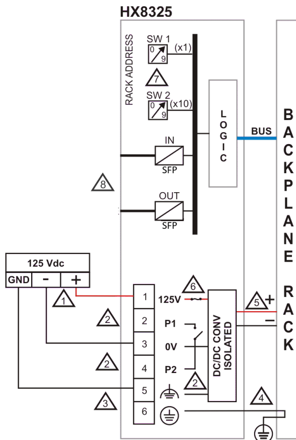
Figura 7: Instalação do Módulo HX8325
