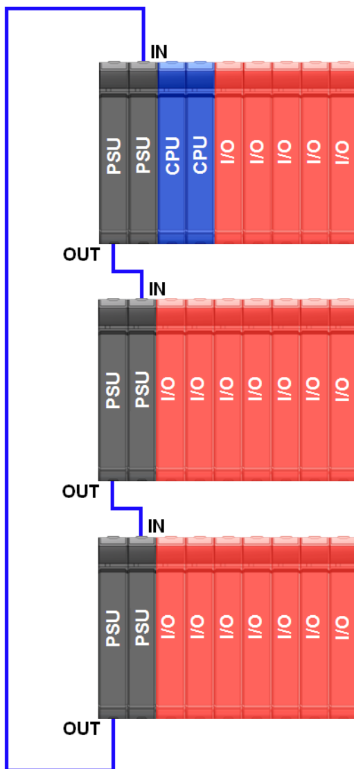
Figura 4: Redundância de Fonte e Expansão de Barramento com Loopback
