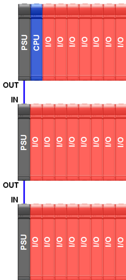
Figura 2: Expansão de Barramento sem Loopback
