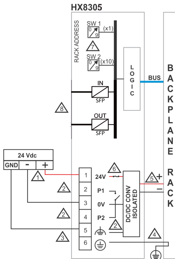
Figura 6: Instalação do Módulo HX8305
